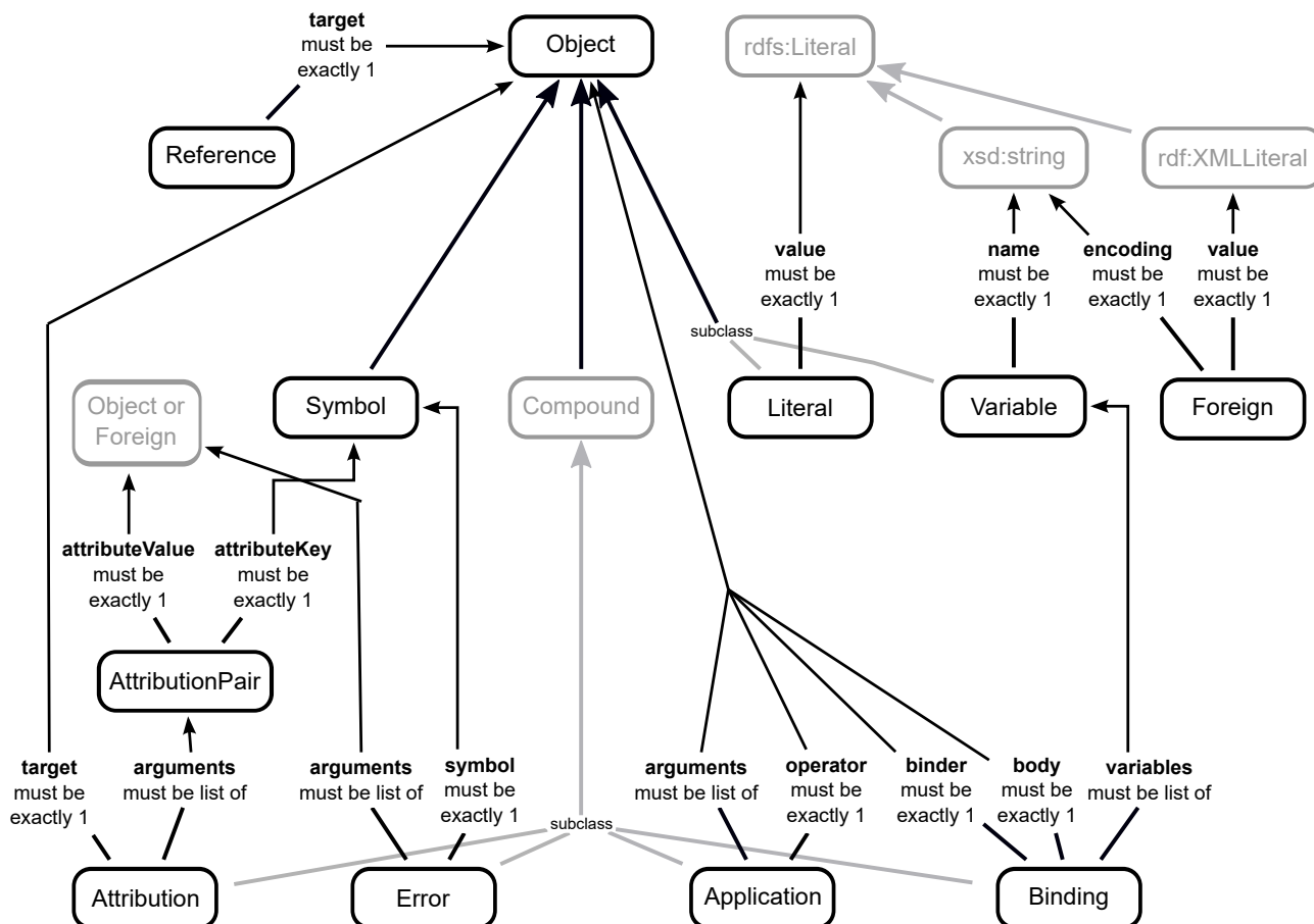
Figure 1: Ontologie für OpenMath-Objekte
