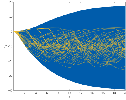
(a) CORA.
