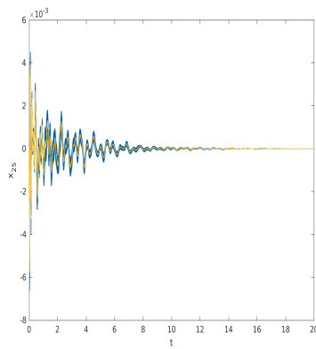
(a) CORA.
